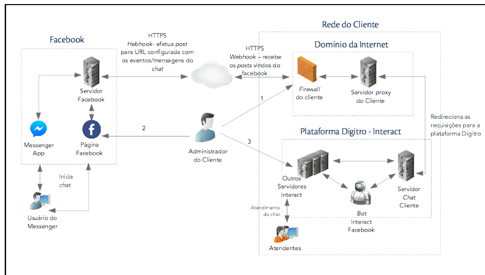
Figura 143. Diagrama – Integração do Interact com o Chat do Facebook Messenger
